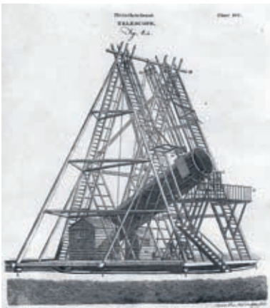
Wilhelm Herschel Teleskop
